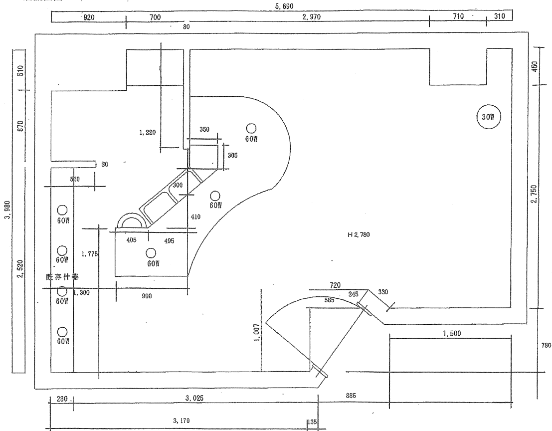
60806 店舗図面
